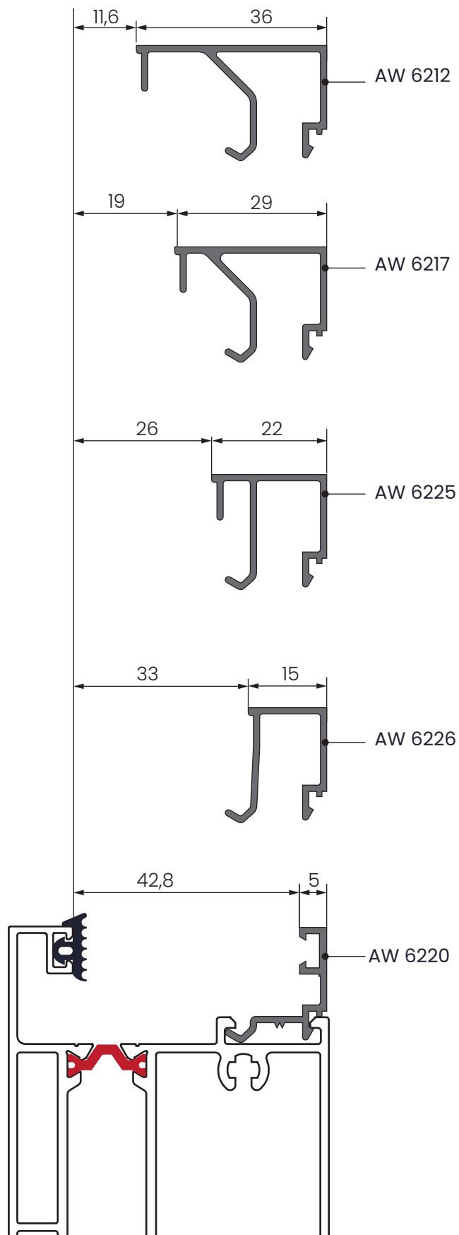
CONTRAVIDRIOS CORTE A 90°
